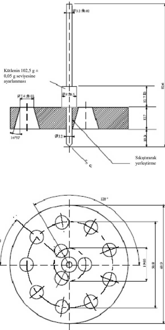
Şekil 1 - Penetrometre
